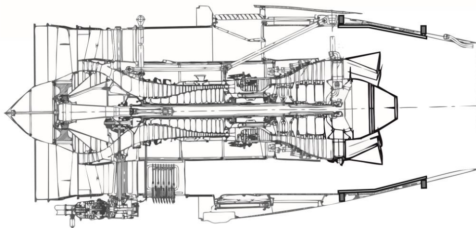
Рисунок 1 – Схема установки предлагаемого устройства в камере смешения ТРДД в исходном положении
