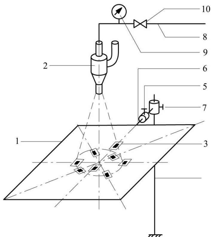
Рис.1 - Общий вид стенда для исследования характеристик воздушной струи с частицами кокса: 1- защитный кожух; 2- эжекторный пистолет; 3- тензо– датчик; 4- стойка; 5- винт; 6- кронштейн; 7- винт; 8- всасывающая магистраль; 9- вакуумметр; 10- дроссель
