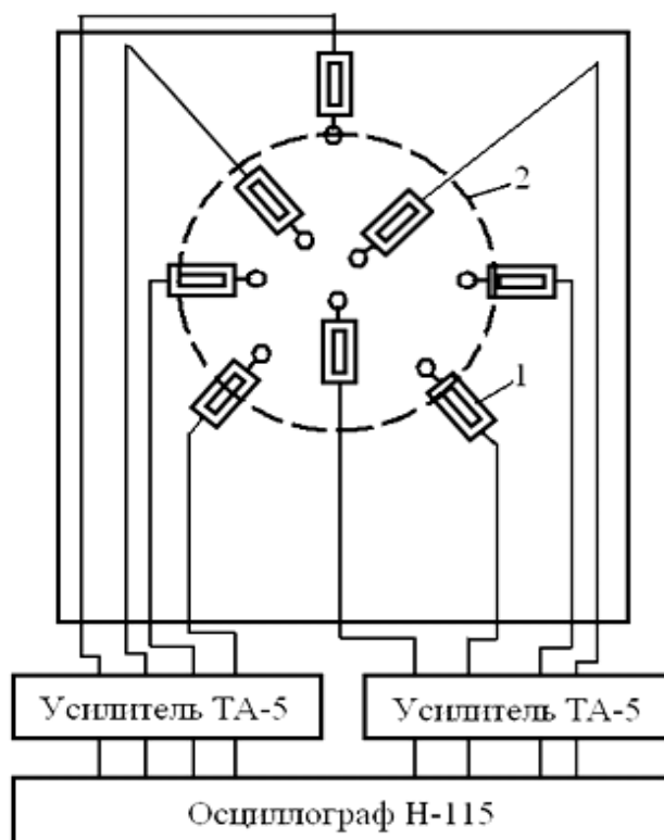
Рис. 2 - Принципиальная схема стенда для исследования характеристик двухфазной турбулентной струи
